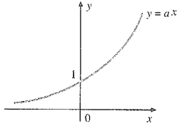
a > 1 için y = a^x in grafiği
